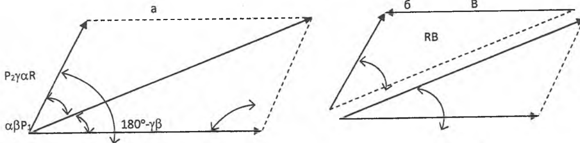
Рисунок 1. Параллелограмм сил
